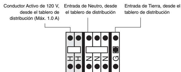
Figura 2 - Alimentación
