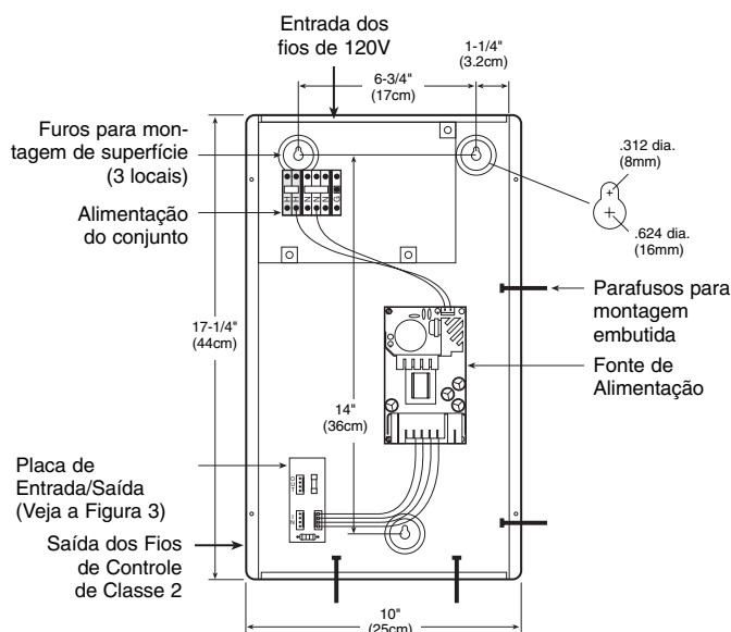
Figura 1 HWI-PS
