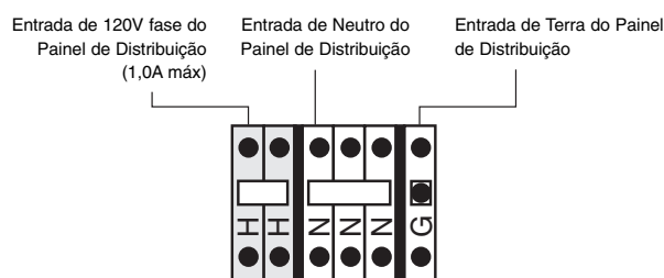
Figura 2 – Alimentação do Conjunto
