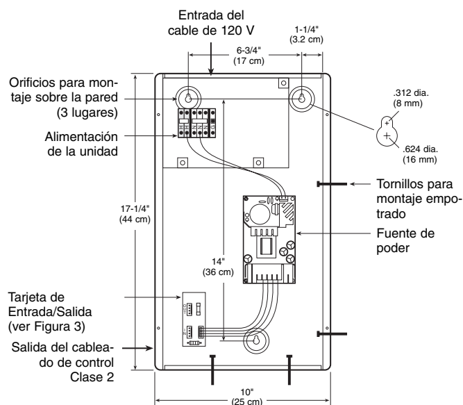
Figura 1 - HWI-PS
