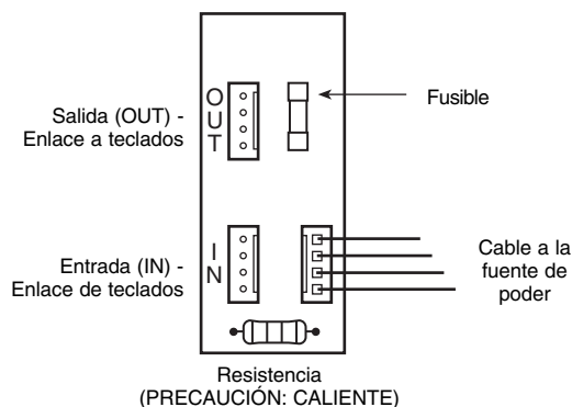
Figura 3 - Tarjeta de Entrada/Salida
