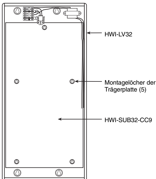
Abbildung 1 - Anordnung der Trägerplatte
