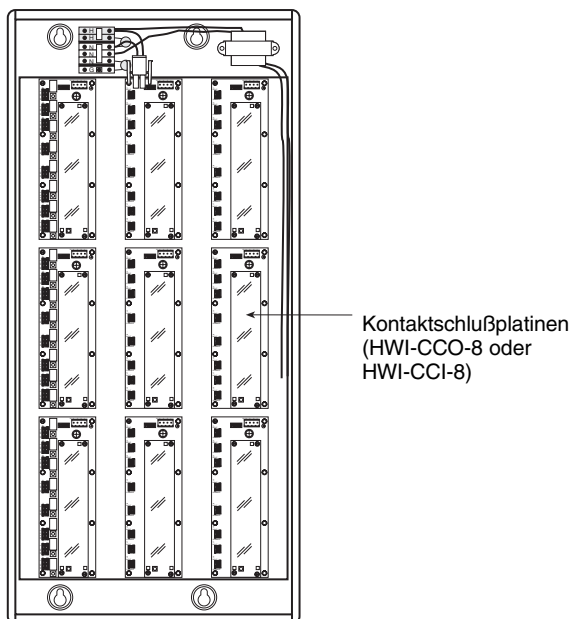
Abbildung 2 - Anordnung der Kontaktschlußplatten
