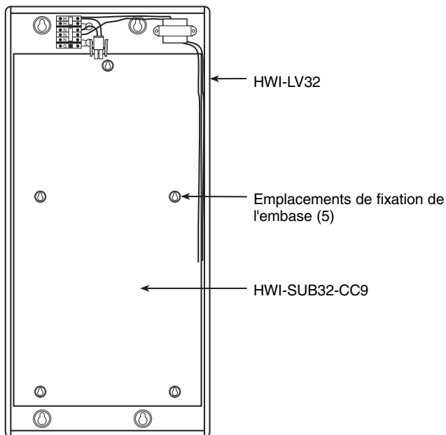
Figure 1 - Emplacement du sous-panneau
