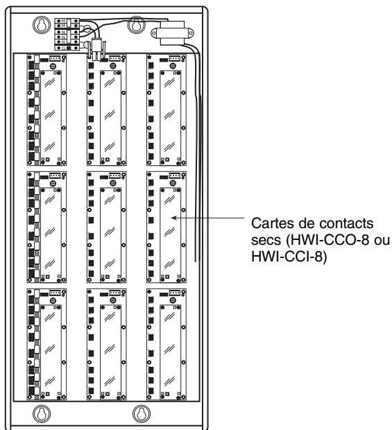
Figure 2 - Emplacement des cartes de fermeture à contact
