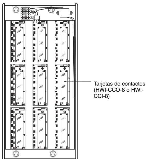
Figura 2 - Posición de las tarjetas de contactos
